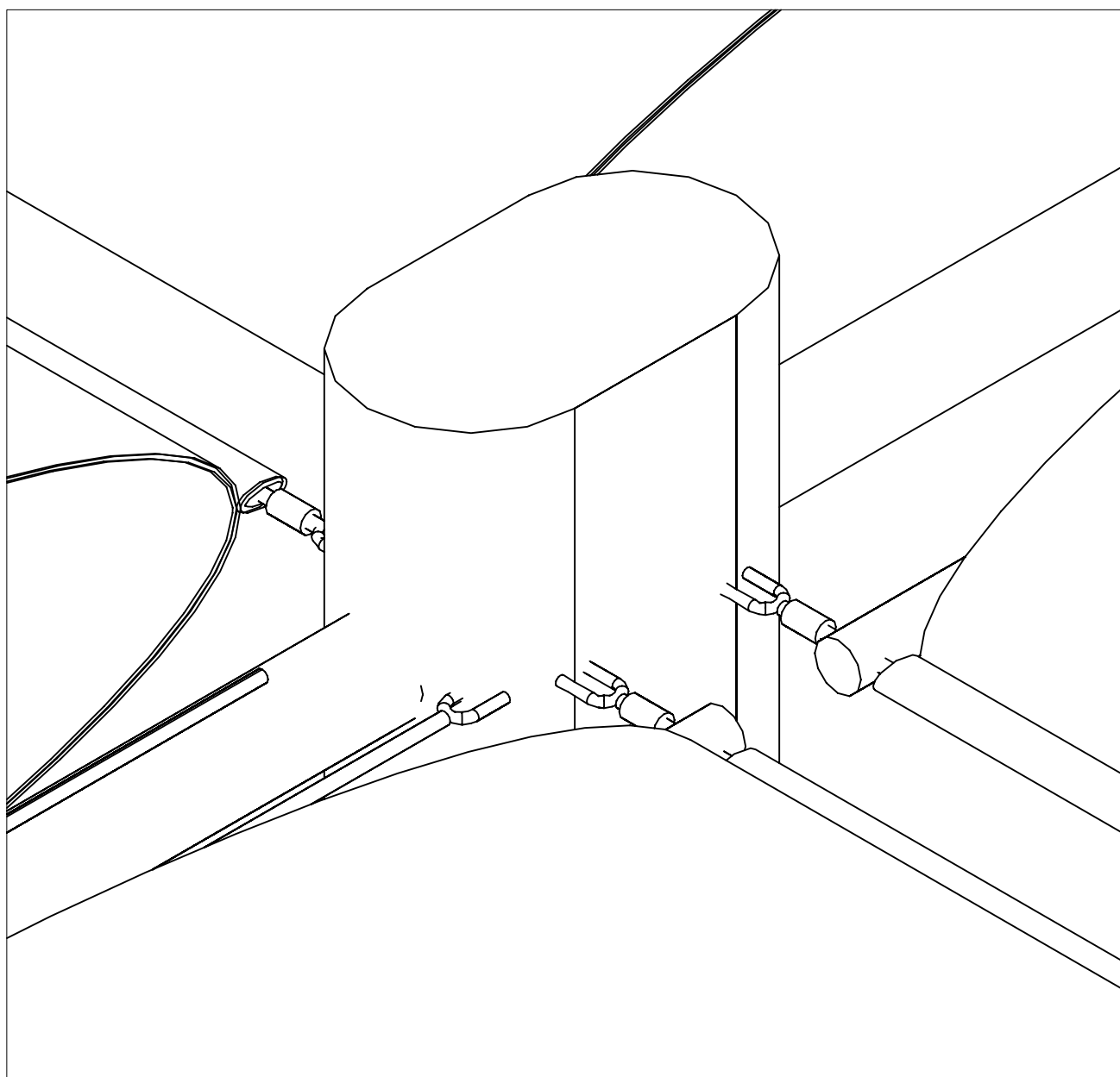
Axonometria de les unions
